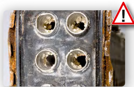
散热器中的水垢
